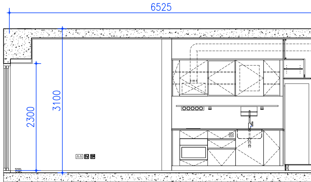
LIV/DIN ELEVATION D1
