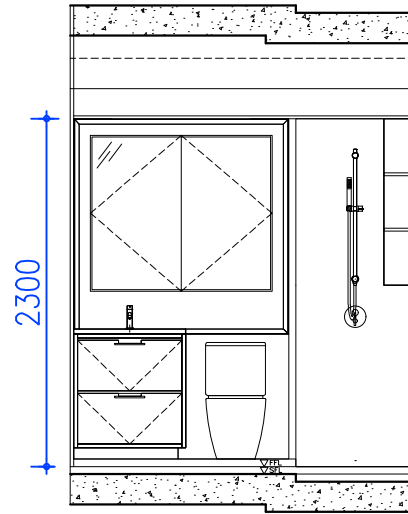
BATHROOM ELEVATION D8
