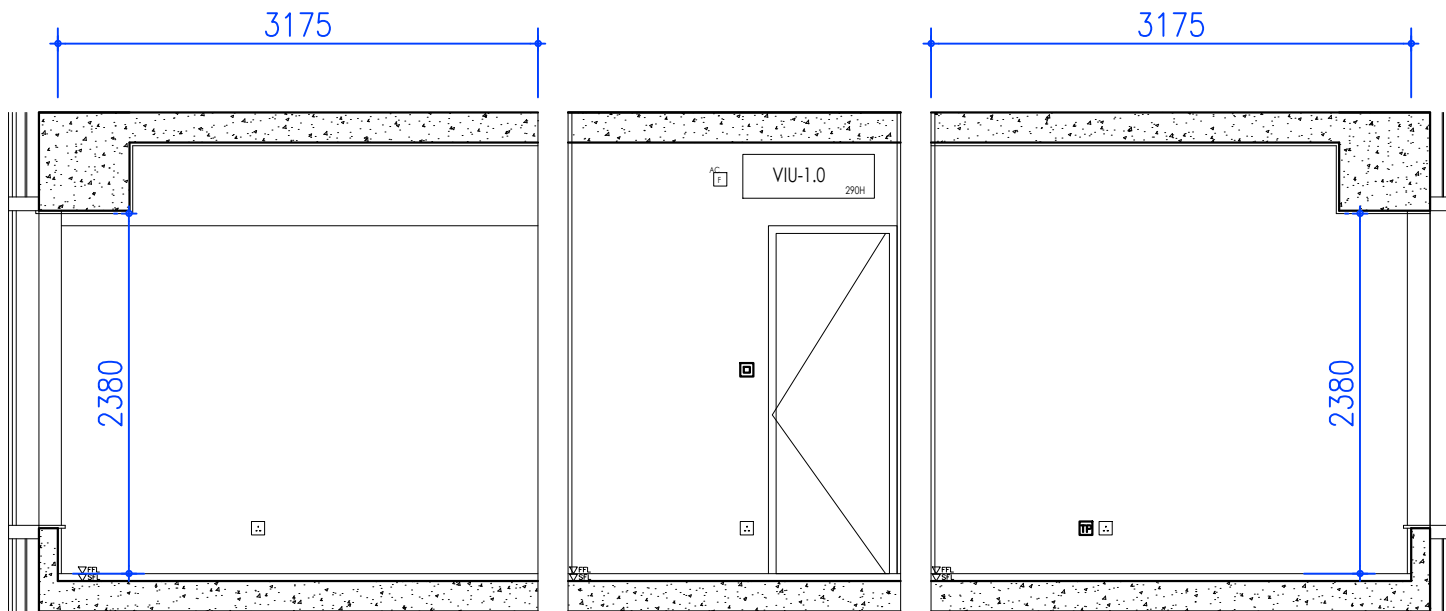
BEDROOM 1 ELEVATION D10
