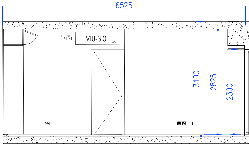
LIV/DIN ELEVATION D3
