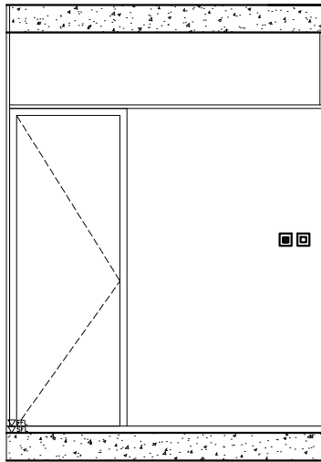
CORRIDOR ELEVATION D7
