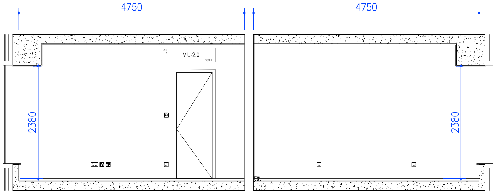
MASTER BEDROOM ELEVATION D13
