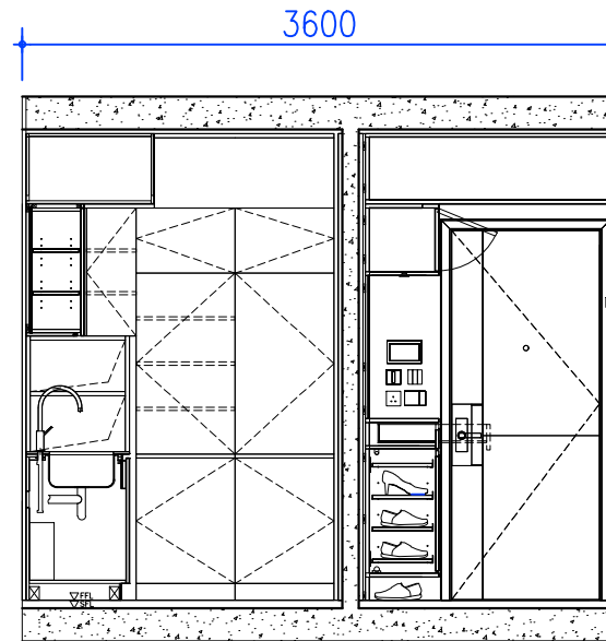
LIV/DIN ELEVATION D2
